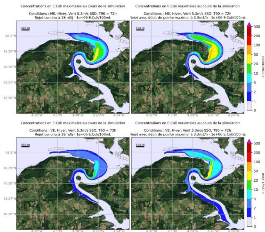
Figure 6-4: Concentrations maximales au cours de la simulation pour les conditions hivernales et une hypothèse de rejet de 1E6E.coli/100mL (ME en haut, VE en bas ; Rejet continu à gauche et rejet avec débit de pointe à droite)
