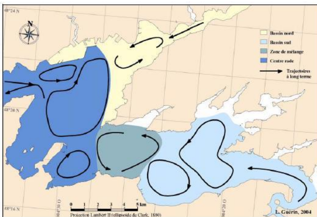
Figure 10 : Délimitation et trajectoire à long terme des principales masses d'eau dans l'hydrosystème rade de Brest (d'après Salomon et Breton, 1991, in Guérin, 1997a, 2004).
