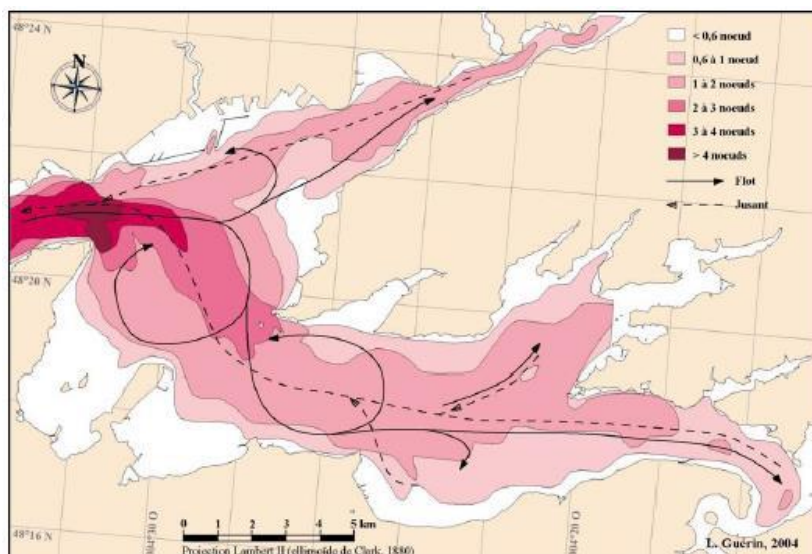
Courants de marée en rade de Brest (coeff. 95) : intensité maximale et circulation au flot et au jusant (d'après S.H.O.M, 1994, in Guérin, 1997a, 2004)
